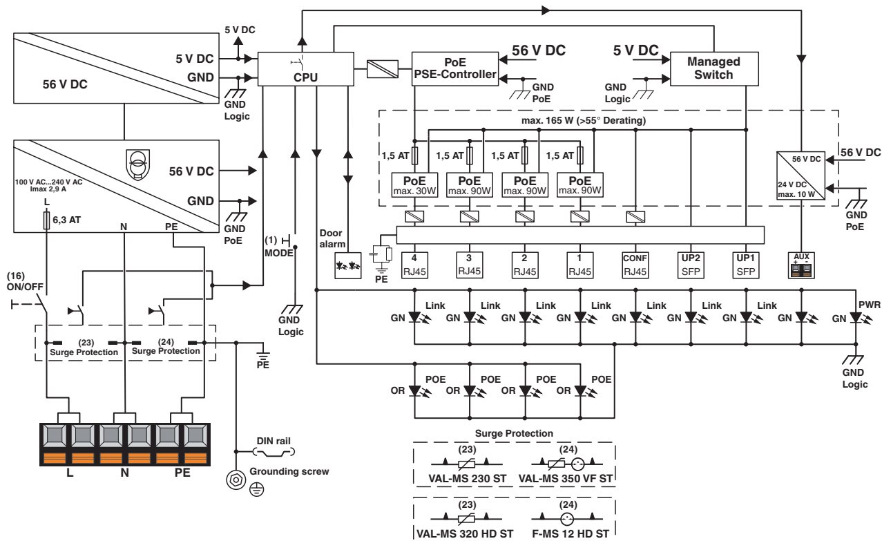
Bild 3 Prinzipschaltbild
